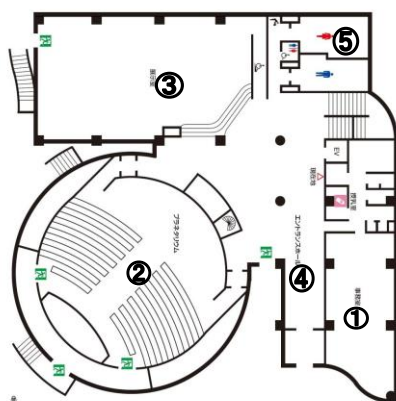
1階平面図
