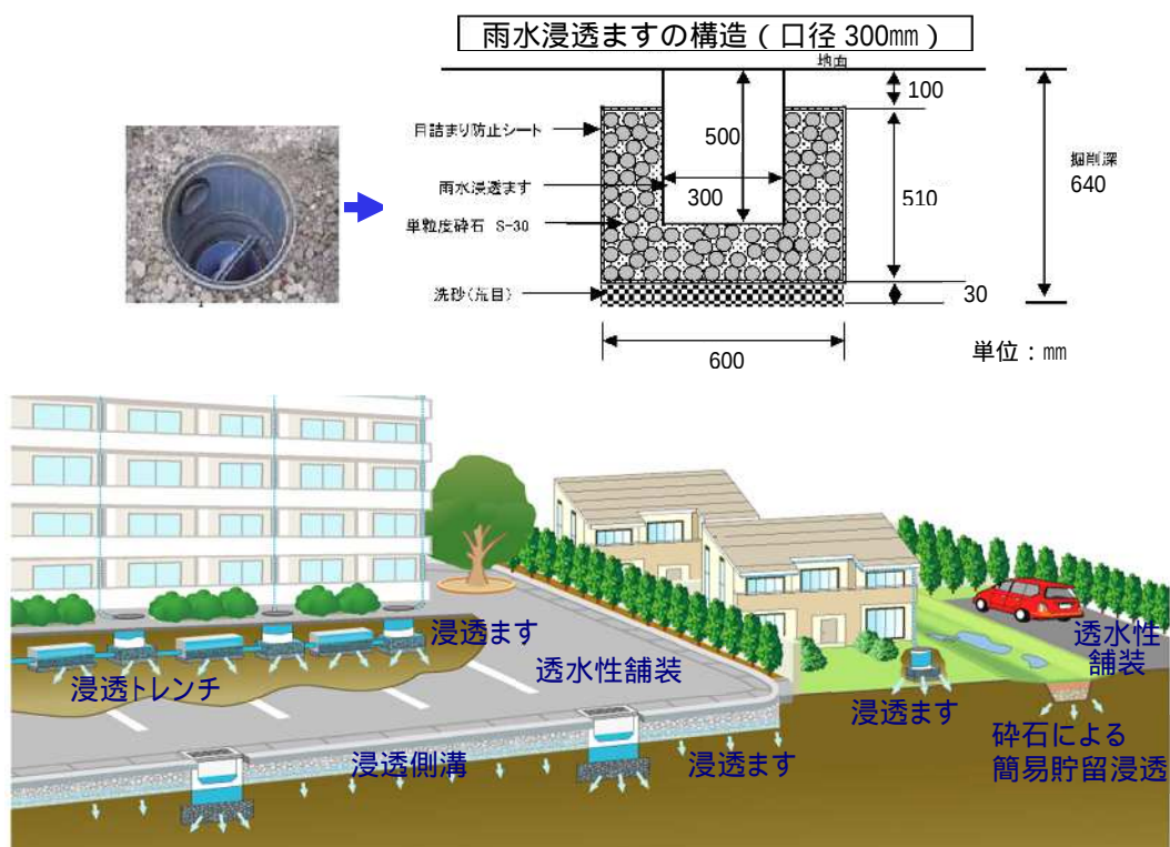
図4-2 雨水浸透施設の設置のイメージ
