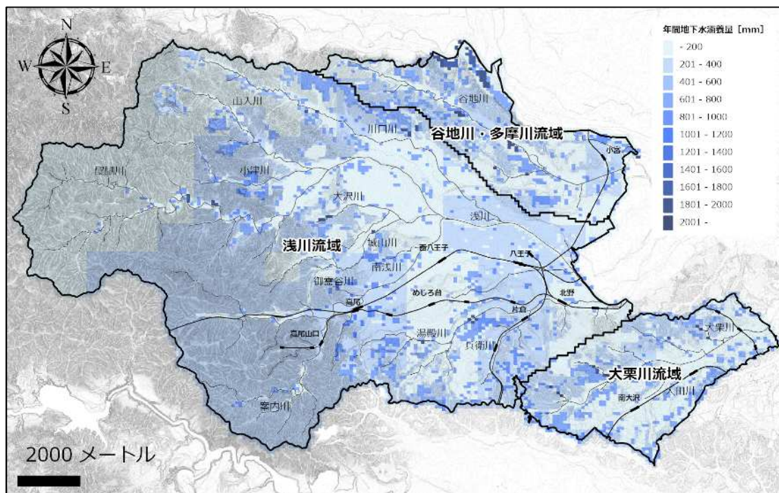
図資-28 八王子市における地下浸透量のイメージ
