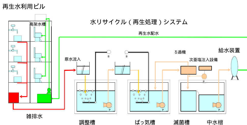
図4-25 南大沢水リサイクルセンターの中水利用
