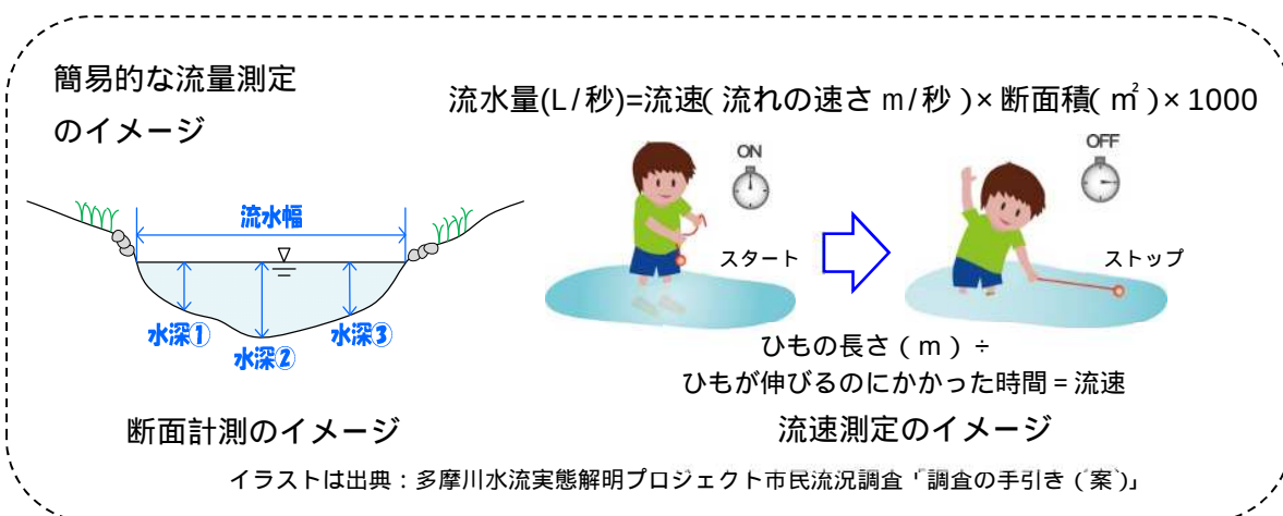
図4-8 河川の簡易的な流量・流速測定イメージ
