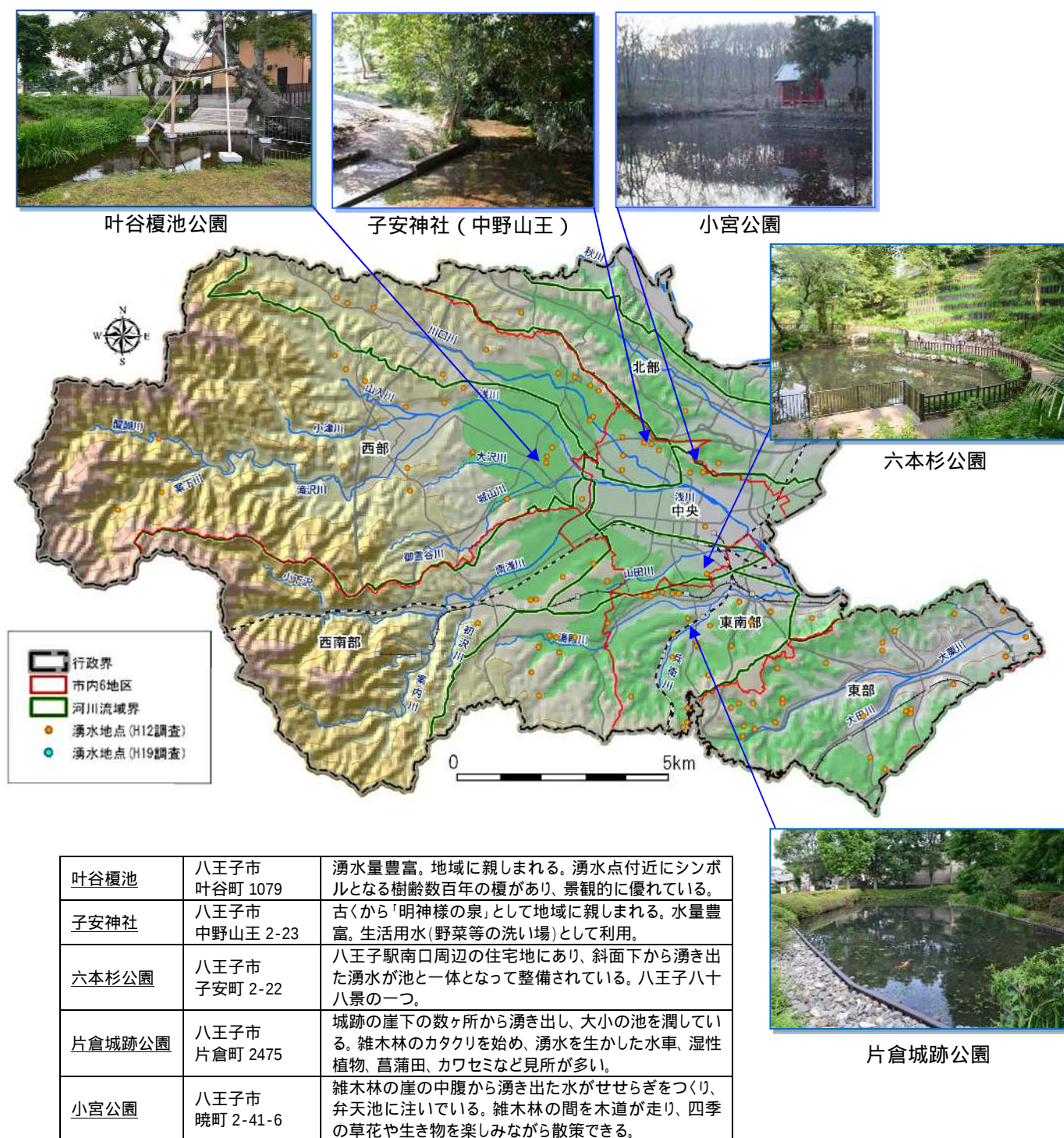
図資-11 八王子市の湧水と東京都の名湧水に選定されている湧水
