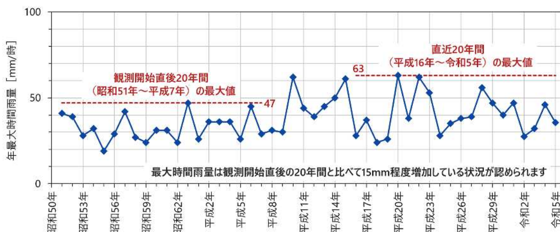
図資-3 年最大時間雨量の変化 (昭和 51 年～令和 5 年) (地域気象観測システム (アメダス))
