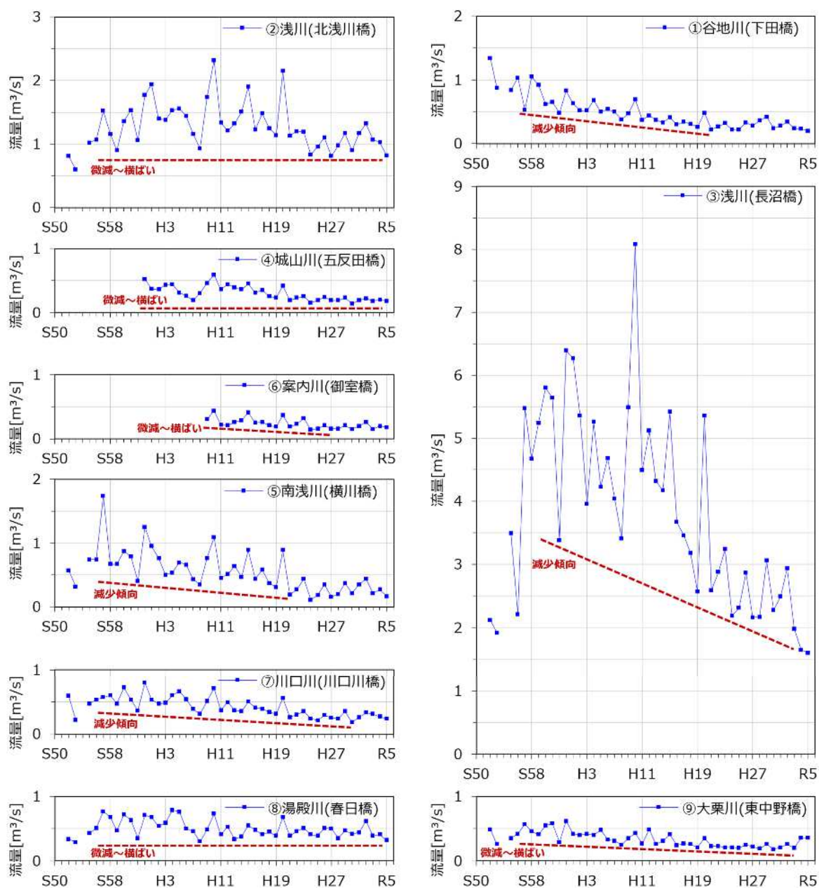
図資-10 河川流量 注 の経年変化
