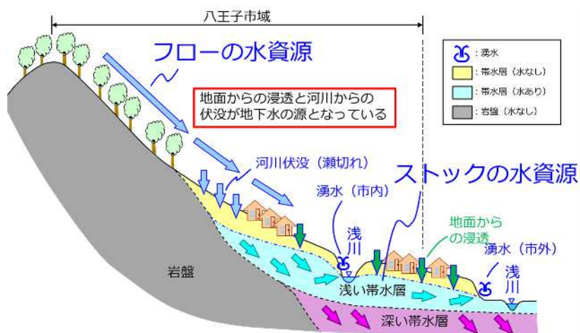
図資-33 八王子における地下水の流動
