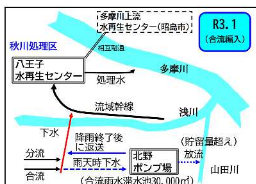
図5-3 流域下水道への編入イメージ
