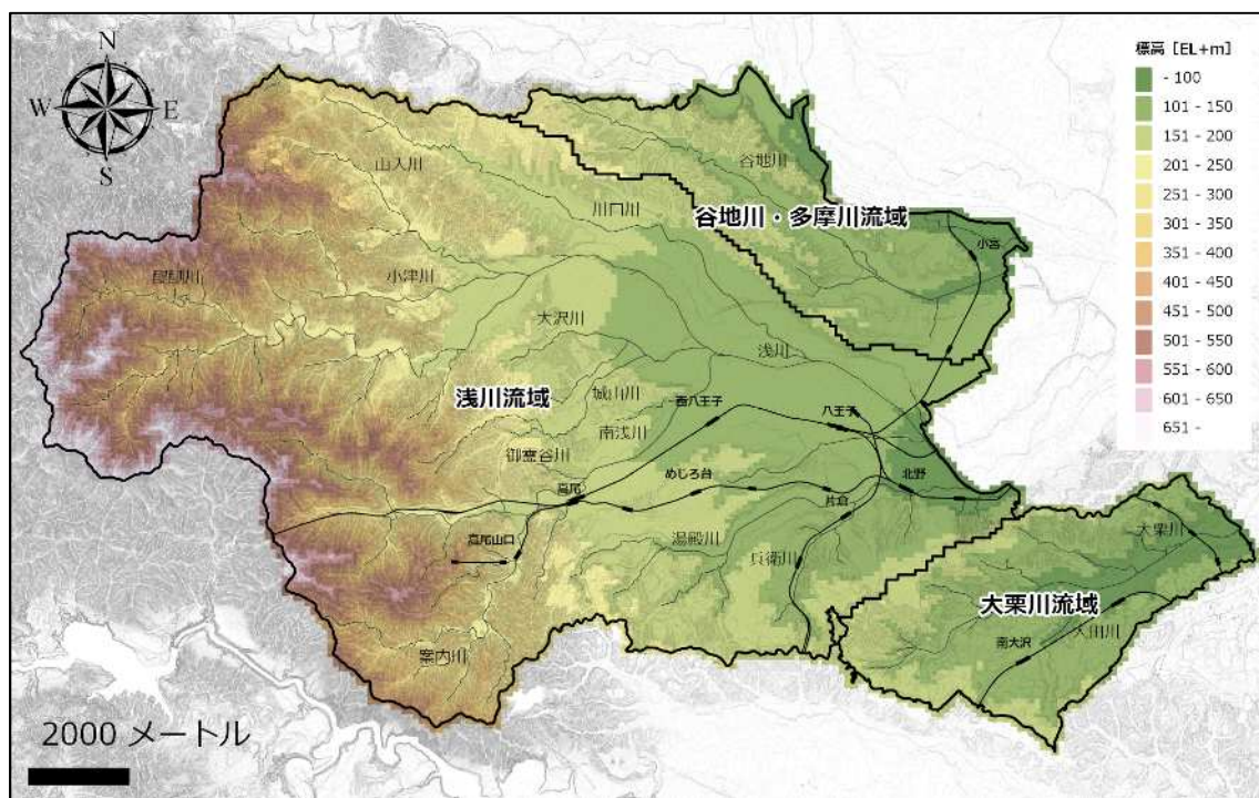
図資-24 八王子市の地形(標高)
