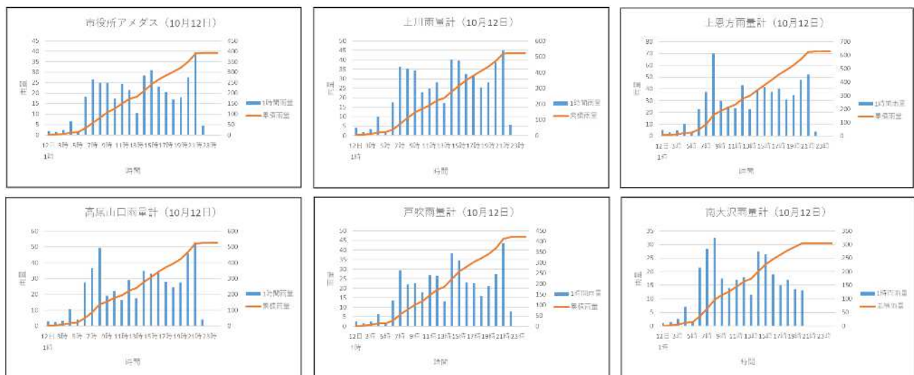
図資 - 1 6 各観測所における降水量の推移 (令和元年 10 月 12 日 0 時 ~ 12 日 24 時)
