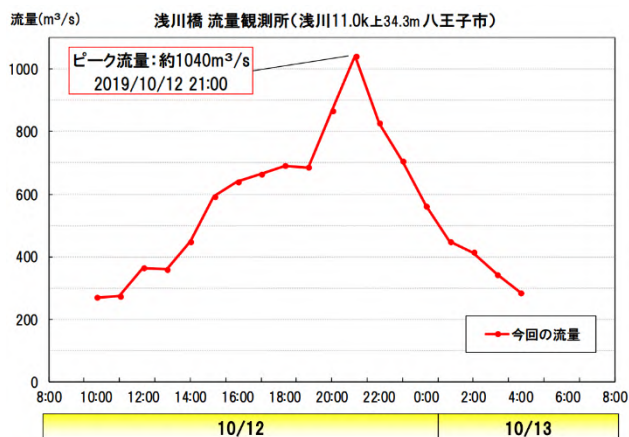
図1-2 令和元年台風19号の降雨による、浅川橋での水量の変化
