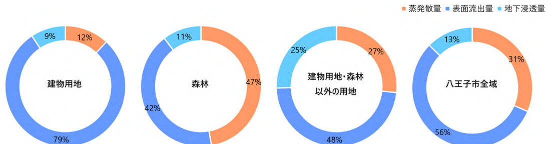
図資-26 八王子市における地下浸透量のイメージ
