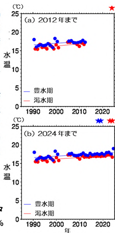
図4-16 子安神社（中野山王）における水温の経年変化
