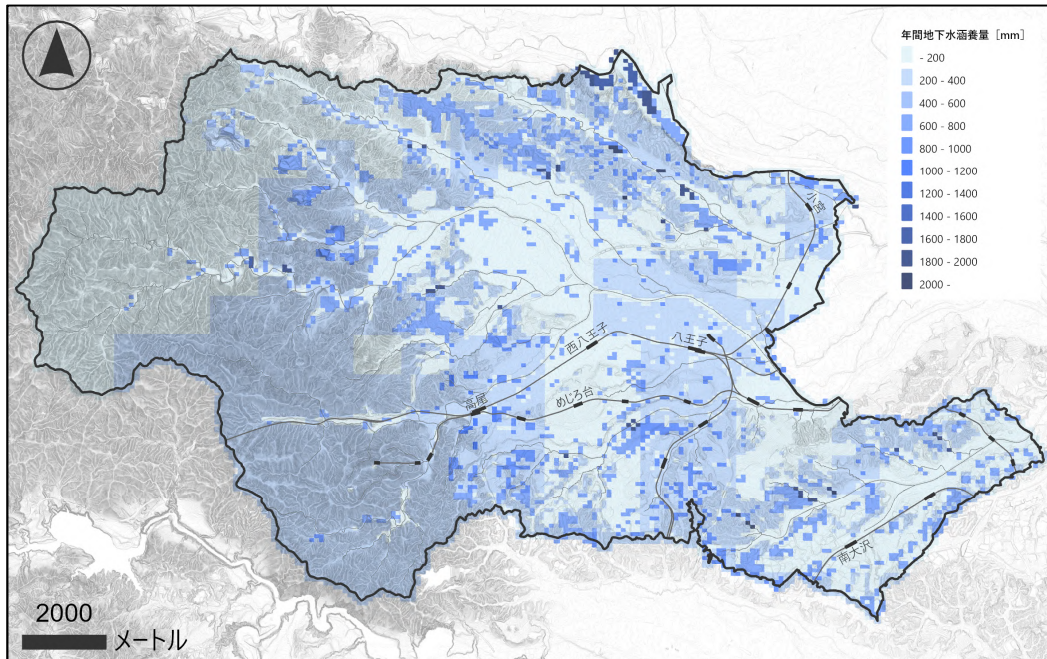
図資-26 八王子市における地下浸透量のイメージ
