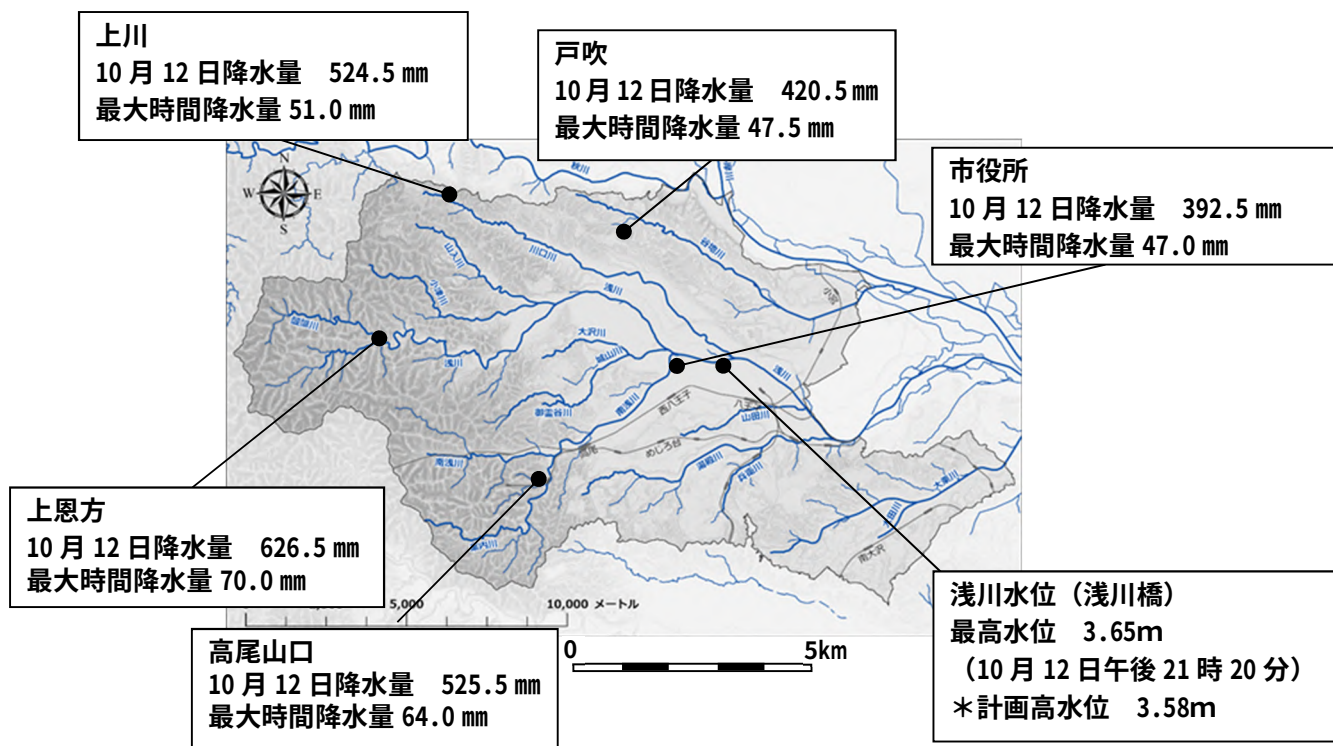
図資-11 令和元年台風第19号における市内の降水量と浅川の水位
