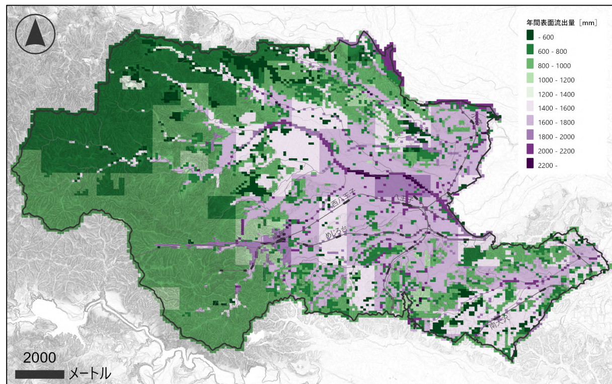
図資-25 八王子市における表面流出量のイメージ
