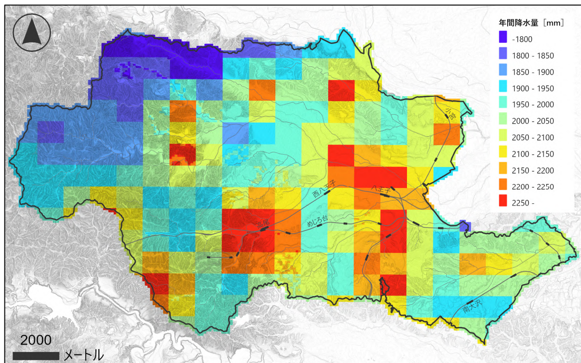
図資-23 八王子市の年間降水量のイメージ（メッシュ平均値 2020）
