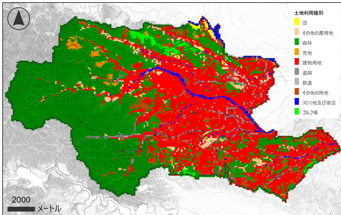
図資-21 八王子市における現在の土地利用
