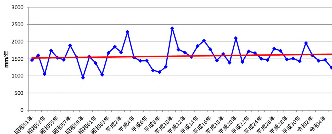
図資-2 年総雨量の変化（昭和 51 年～令和 5 年） （地域気象観測システム（アメダス））
