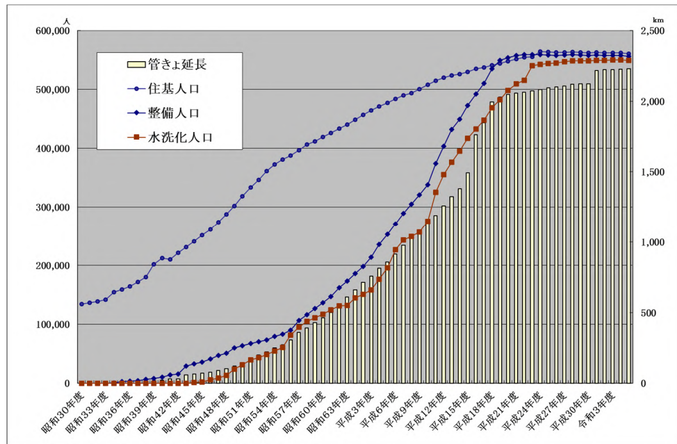
図資-16 公共下水道の管きょ延長と整備人口・水洗化人口の推移
