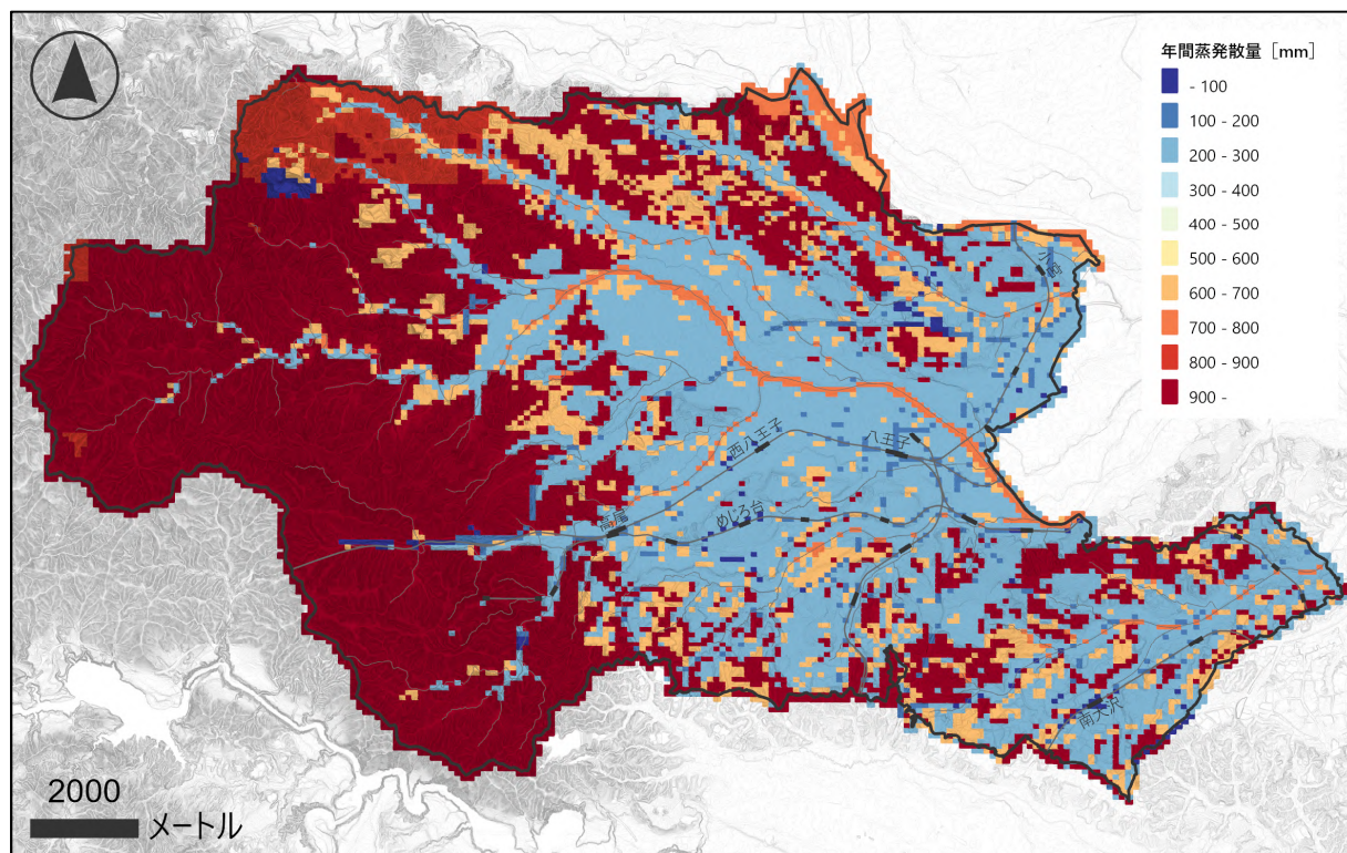
図資-24 八王子市における蒸発散量のイメージ
