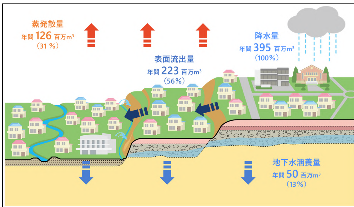
図資-27 八王子市全域の水収支のイメージ
