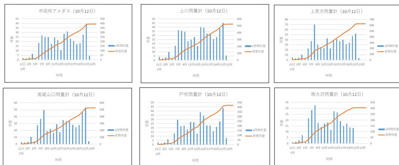
図資-12 各観測所における降水量の推移 (令和元年10月12日0時～12日24時)
