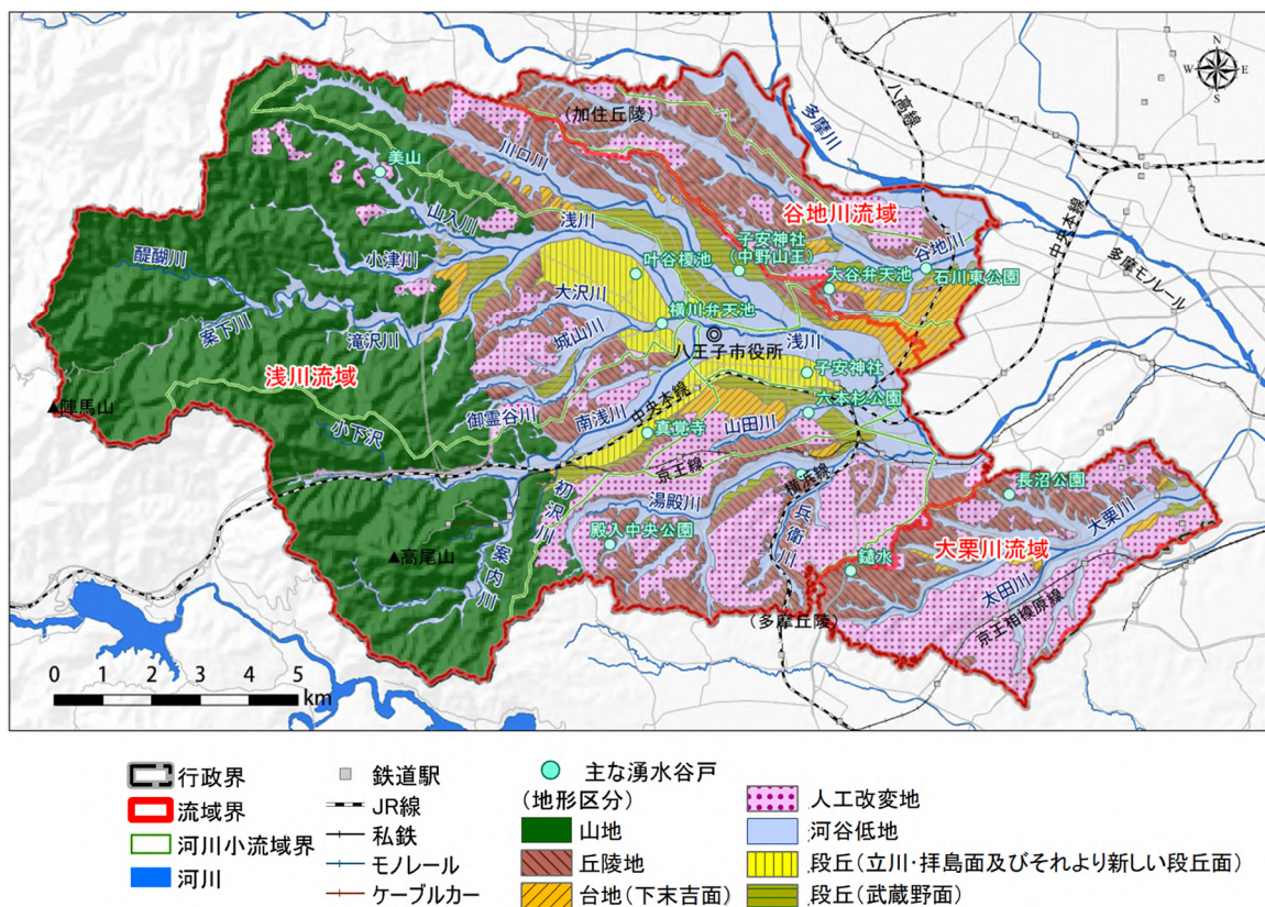
図2-6 計画の対象範囲（八王子市の地形）
