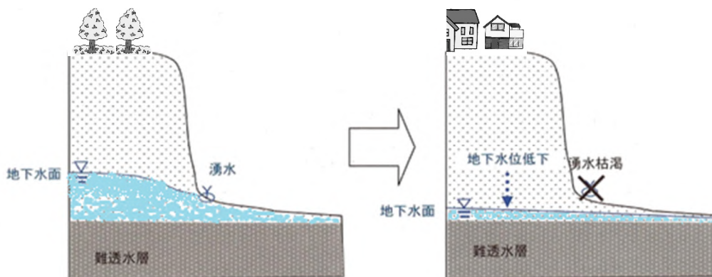
図1-1 土地利用の変化による湧水の枯渇や地下水位低下のイメージ
