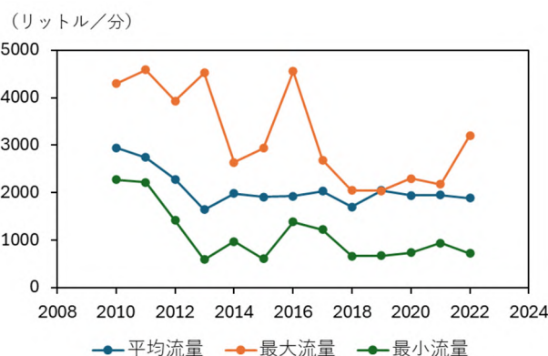
図4-15 子安神社（中野山王）における湧水量
