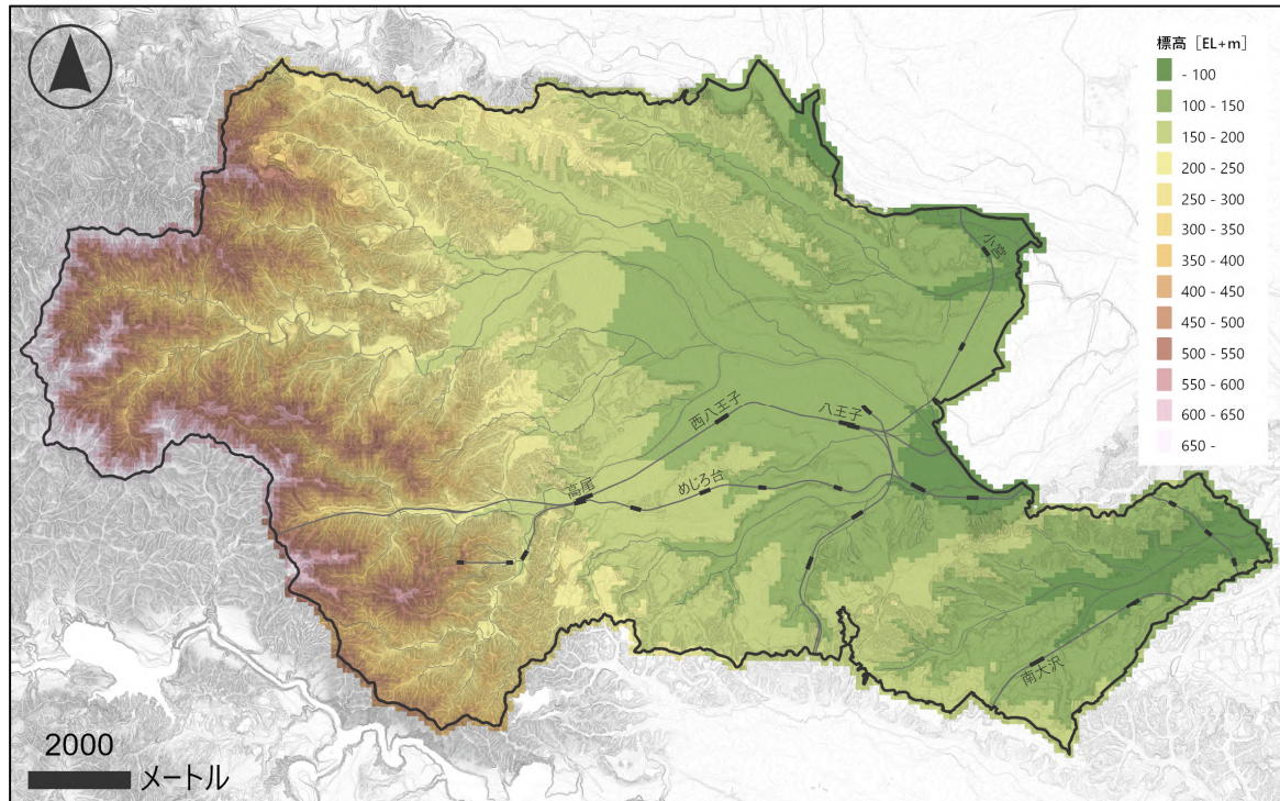
図資-22 八王子市の地形（標高）
