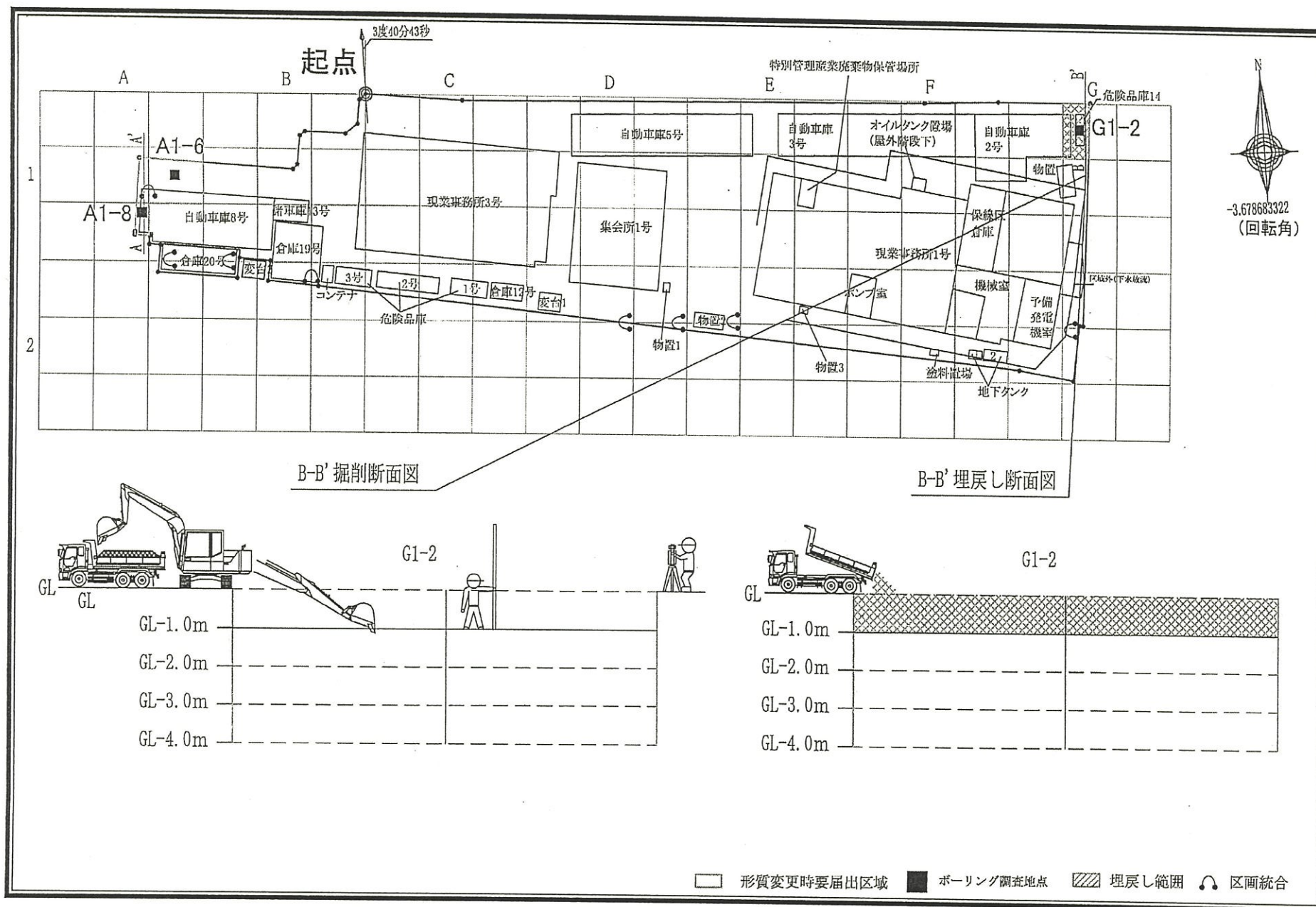
図-3-2 措置対策施工平面・断面図 (G1-2 区画)
